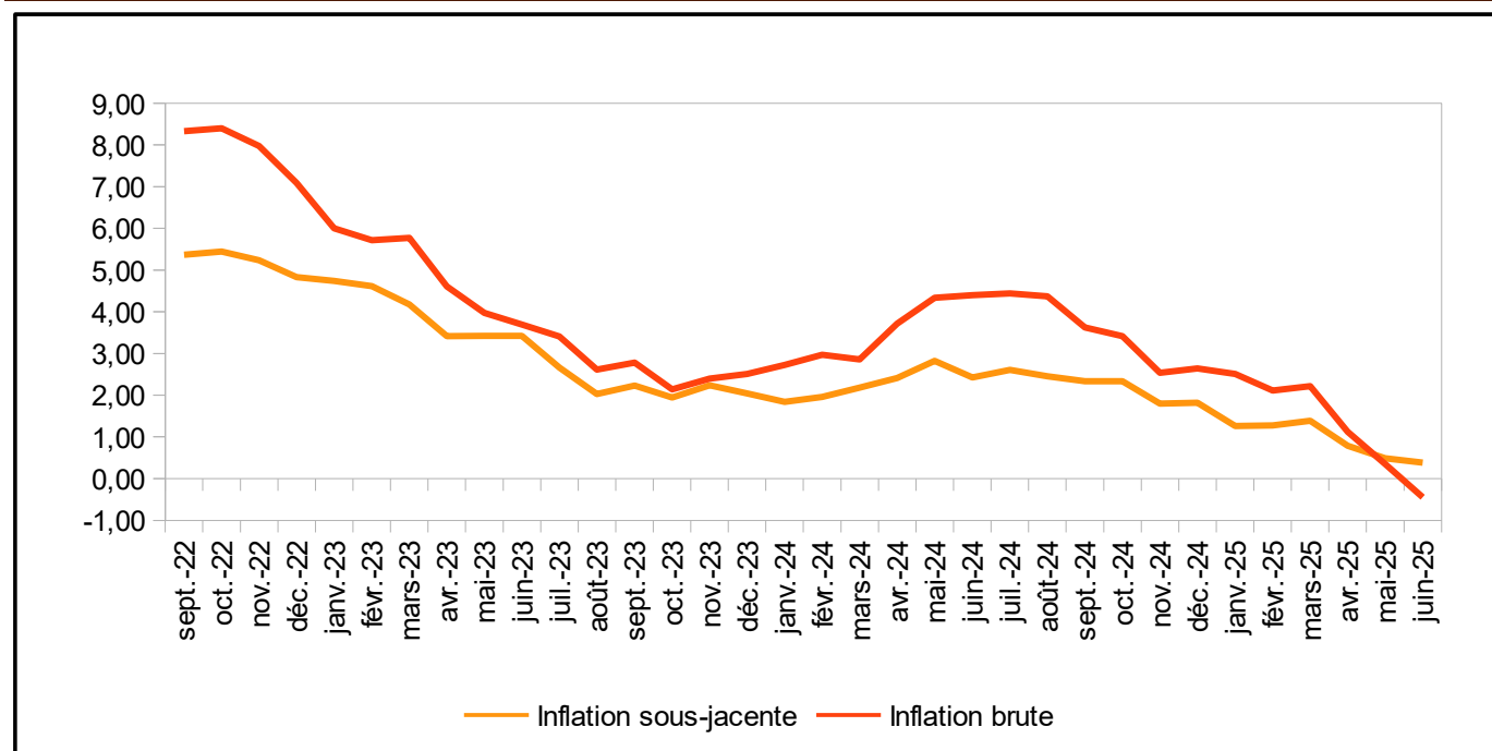
Graphique 11.1 Evolution de l'IHPC et de l'inflation sous-jacente dans l'UEMOA (Glissements annuels en pourcentage)
