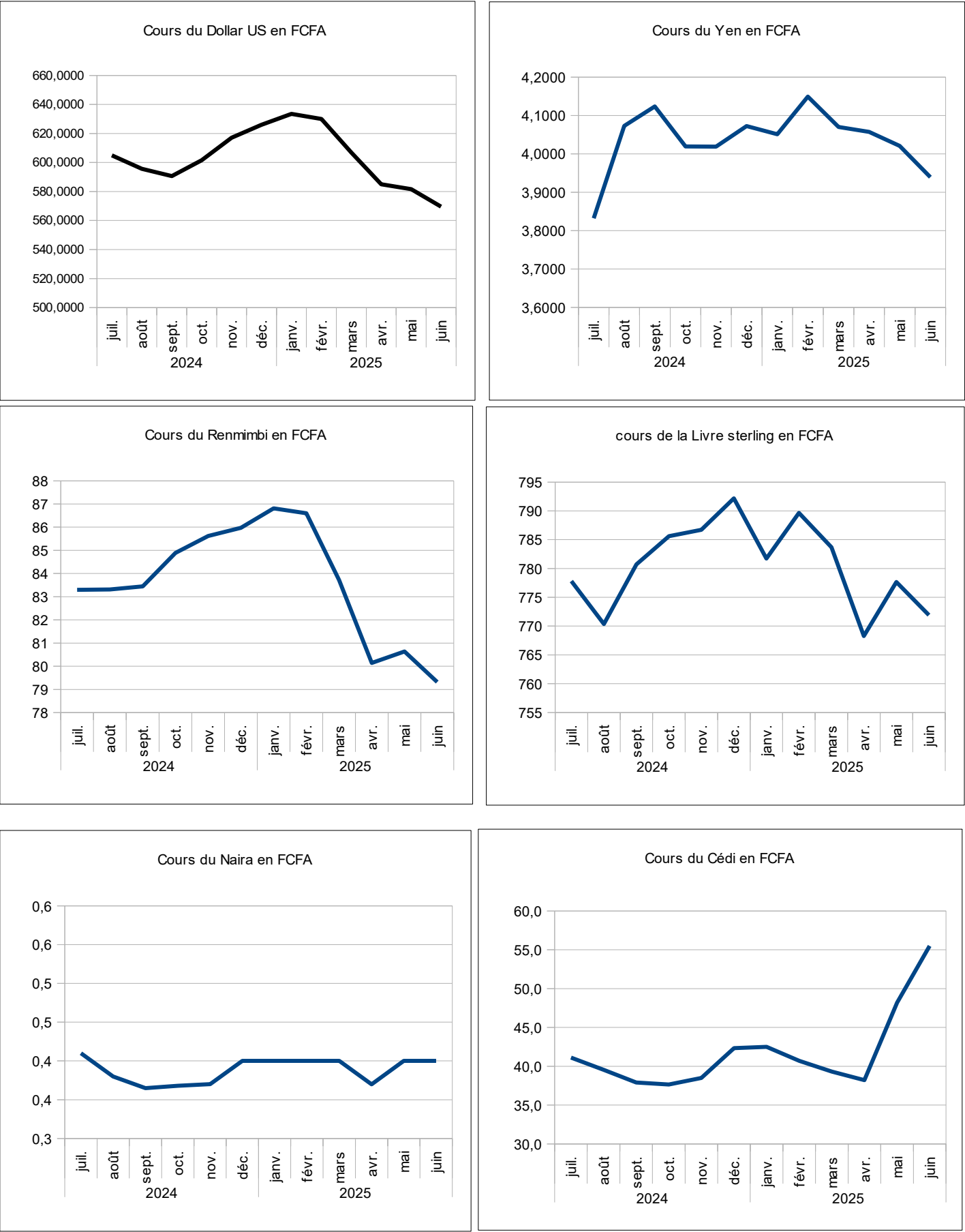
Graphique 9.2 Taux de change bilatéraux (valeur moyenne sur la période : unités de FCFA pour une unité de monnaie étrangère)
